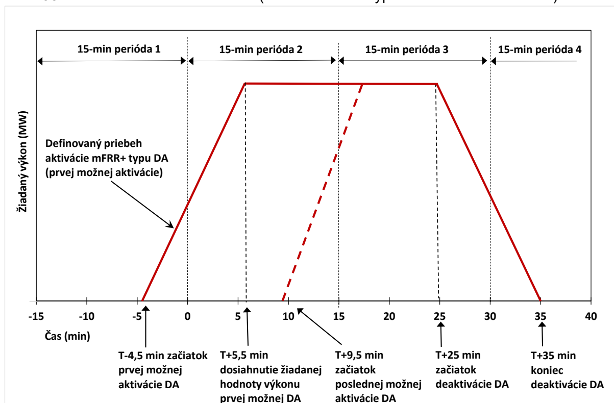
Obr. B4.2 Definovaný priebeh aktivácie typu DA
