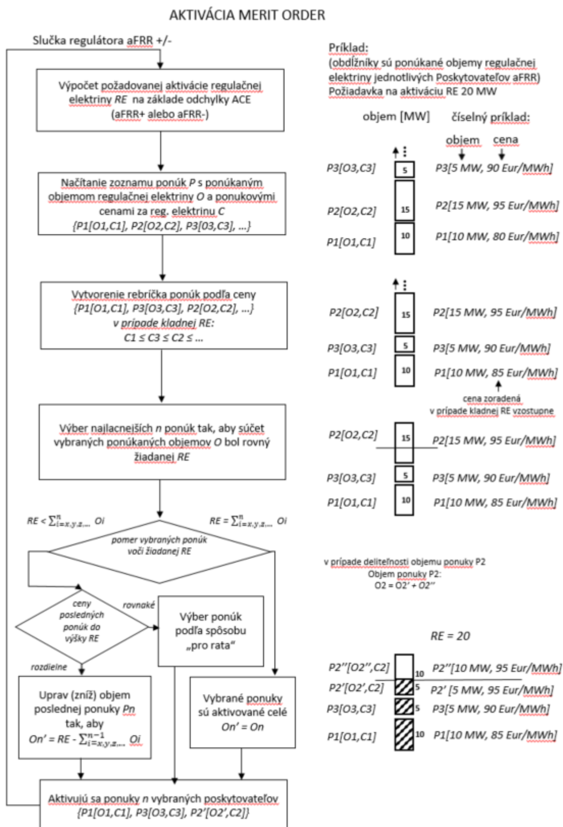
Obr. B2.5 Proces prerozdelenia žiadaného výkonu v aFRR+/aFRR- (Merit order)
