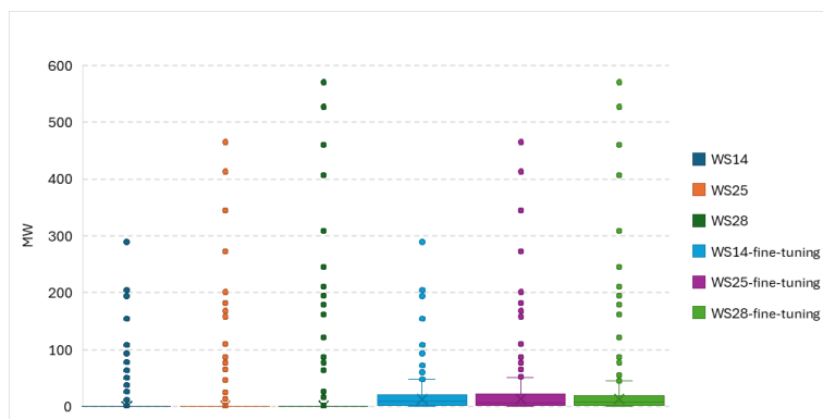
Obr. č. 5.1.1.2_9 Pravdepodobnostné rozdelenie celkového obmedzenia výroby z OZE pre rok 2035 pred a po fine-tuningu
