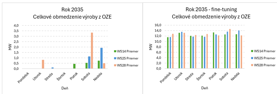
Obr. č. 5.1.1.2_3 Priemerné celkové obmedzenie výroby z OZE v jednotlivých dňoch pre rok 2035 pred a po fine-tuningu
