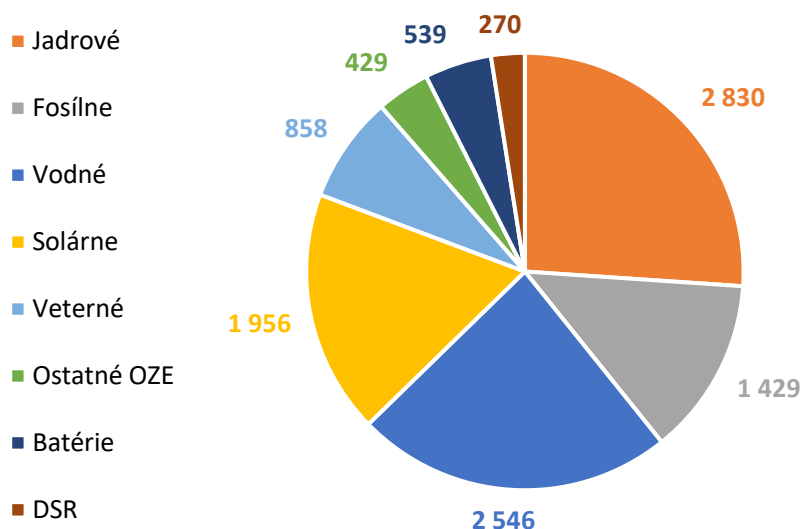
Obr. č. 4.1_2 Čistý inštalovaný výkon zdrojov pre rok 2035
