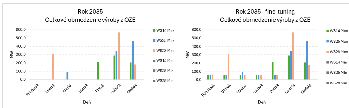
Obr. č. 5.1.1.2_4 Maximálne a minimálne celkové obmedzenie výroby z OZE v jednotlivých dňoch pre rok 2035 pred a po fine-tuningu (Poznámka: WS14-WS28 Min = 0 MW)
