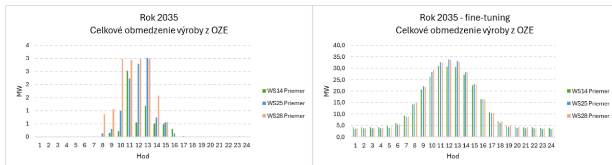
Obr. č. 5.1.1.2_5 Priemerné celkové obmedzenie výroby z OZE v hodinách pre rok 2035 pred a po fine-tuningu
