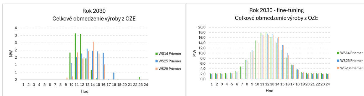
Obr. č. 5.1.1.1_5 Priemerné celkové obmedzenie výroby z OZE v hodinách pre rok 2030 pred a po fine-tuningu
