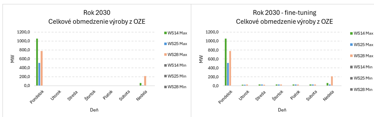
Obr. č. 5.1.1.1_4 Maximálne a minimálne celkové obmedzenie výroby z OZE v jednotlivých dňoch pre rok 2030 pred a po fine-tuningu (Poznámka: WS14 - WS28 Min = 0 MW)
