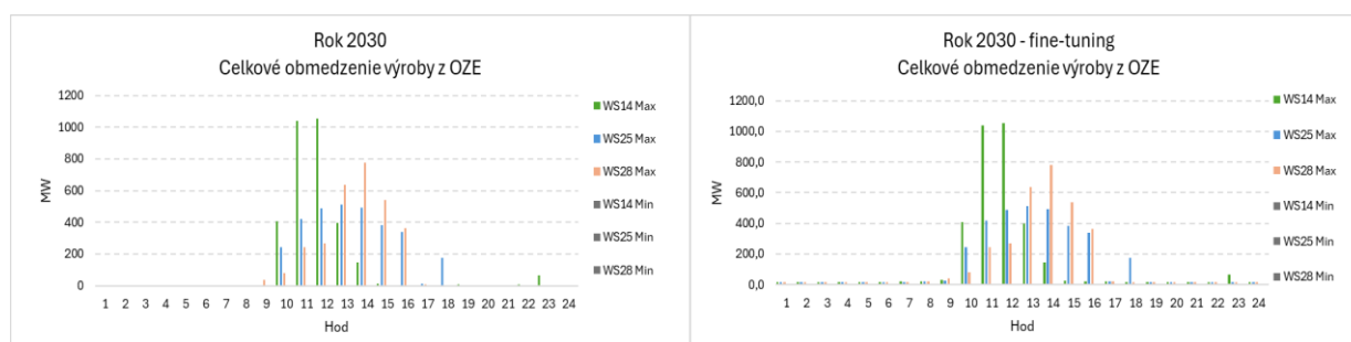
Obr. č. 5.1.1.1_6 Maximálne a minimálne celkové obmedzenie výroby z OZE v hodinách pre rok 2030 pred a po fine-tuningu (Poznámka: WS14 - WS28 Min = 0 MW)
