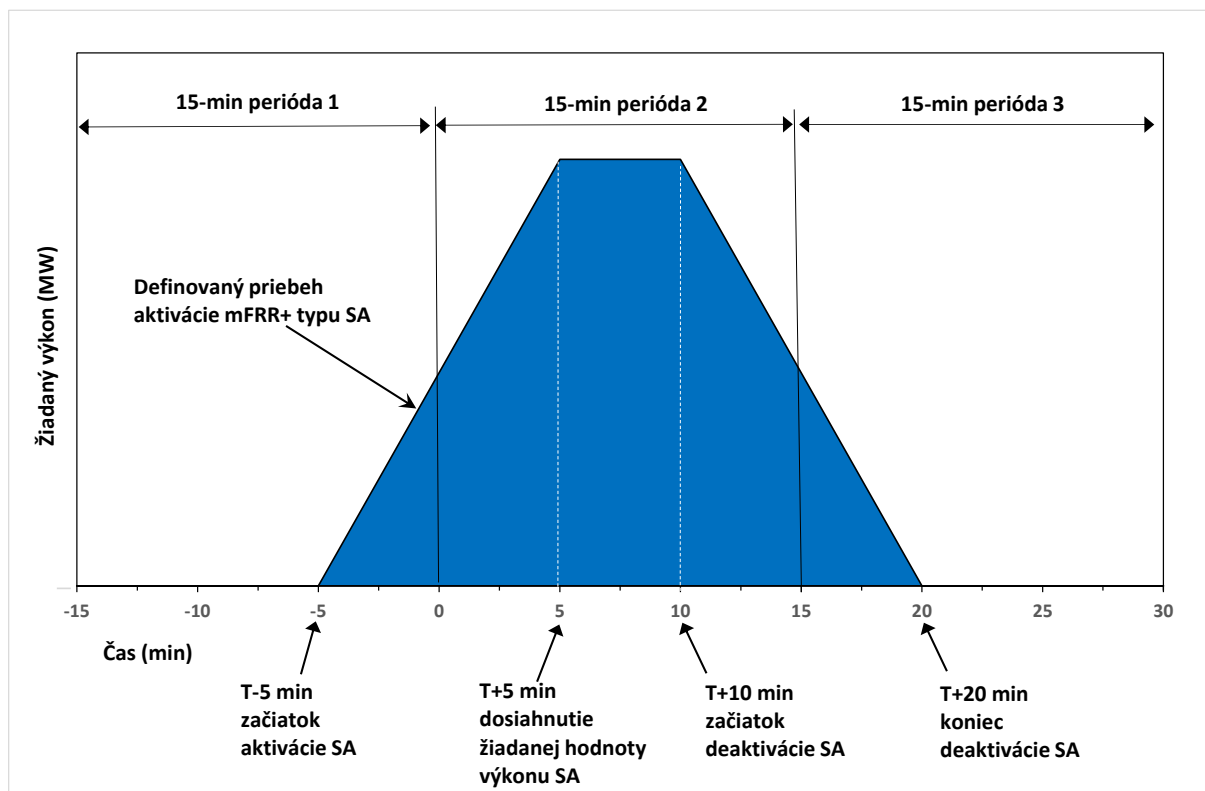
Obr. B4.1 Definovaný priebeh aktivácie typu SA
