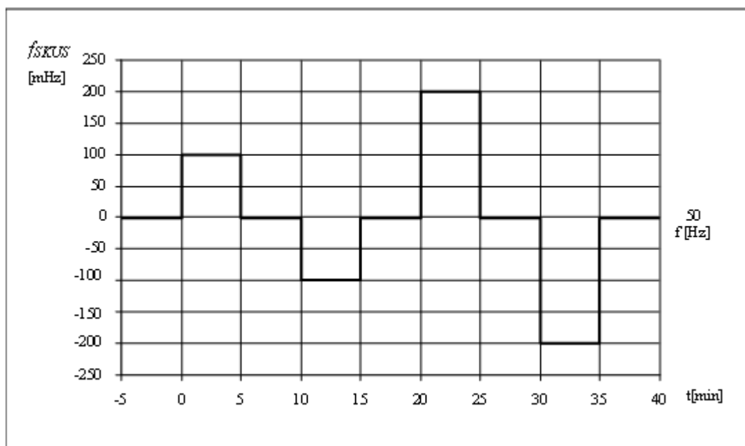
Obr. B5.1 Skúšobný signál pre overenie akčieschopnosti FCR
