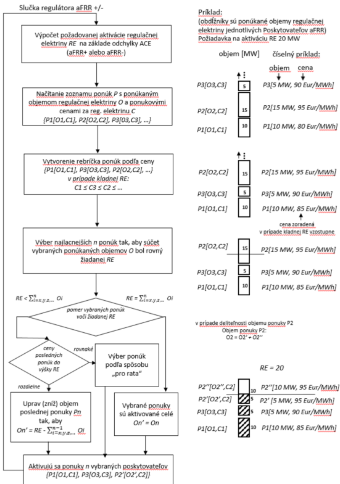
Obr. B2.5 Proces prerozdelenia žiadaného výkonu v aFRR+/aFRR- (Merit order)
